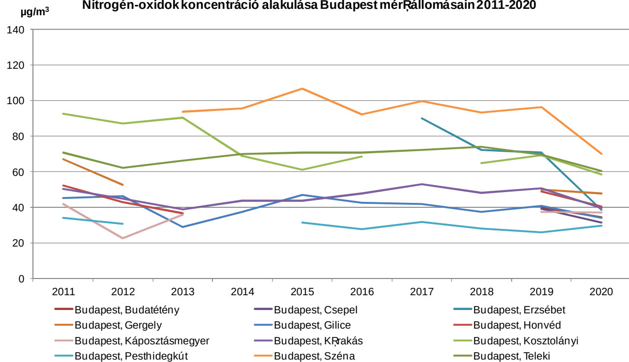
Nitrogén-oxidok koncentráció alakulása Budapest mérőállomásain 2011-2020
