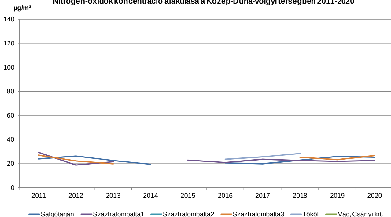
Nitrogén-oxidok koncentráció alakulása a Közép-Duna-völgyi térségben 2011-2020
